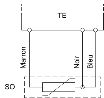
Branchement de la sonde au thermostat electronique
